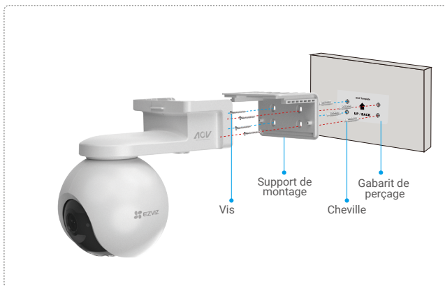
Fig. 2 Montage mural
