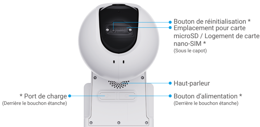
Vue Inférieure
